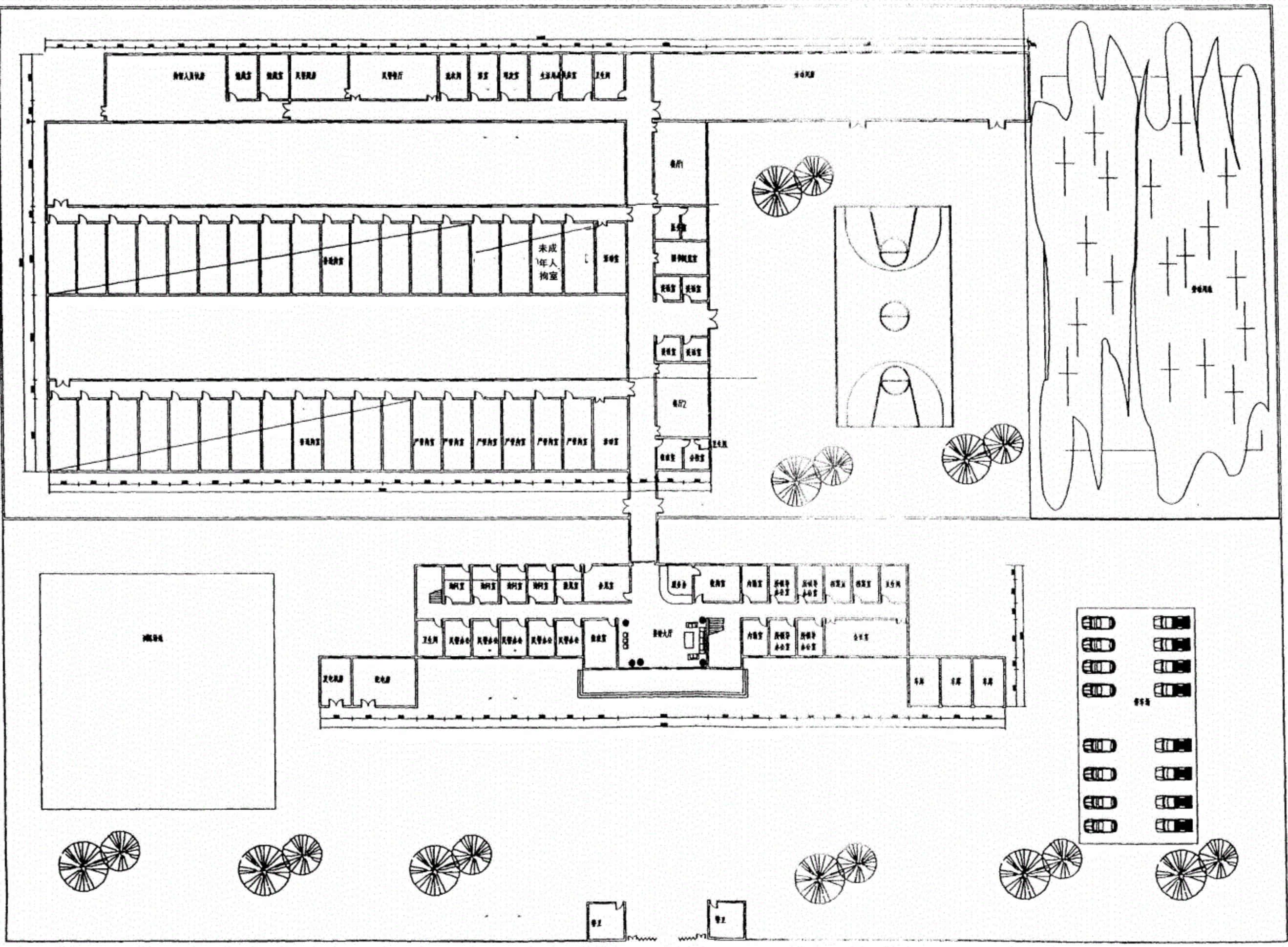
大型、特大型拘留所平面布置示意图
