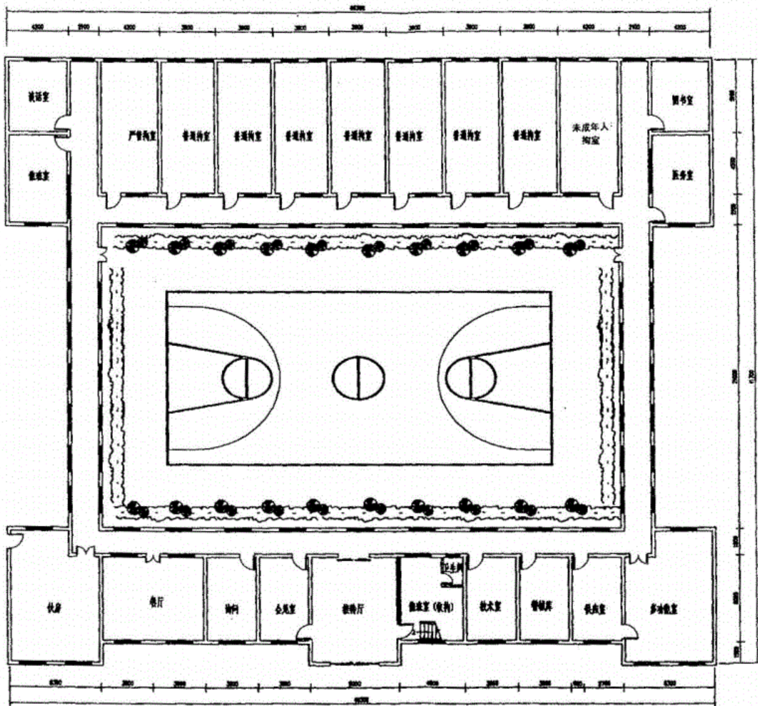
小型拘留所平面布置示意图
