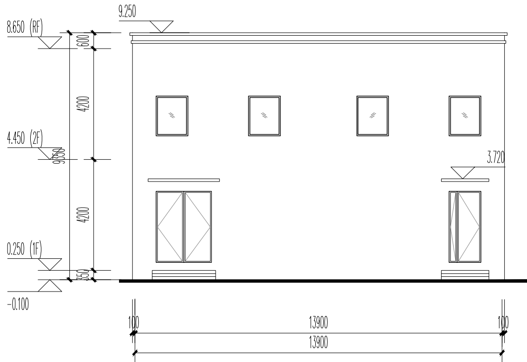
①~③立面图
