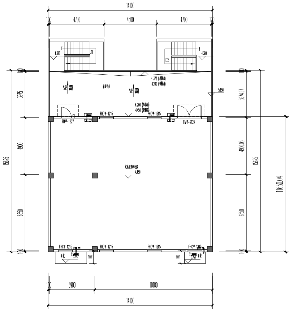
14#楼二层平面图
