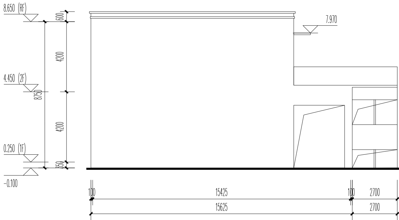
④~①轴立面图
