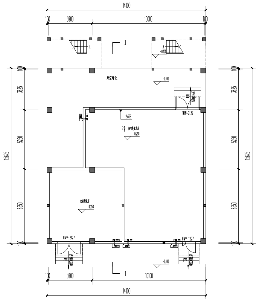
14#楼一层平面图
