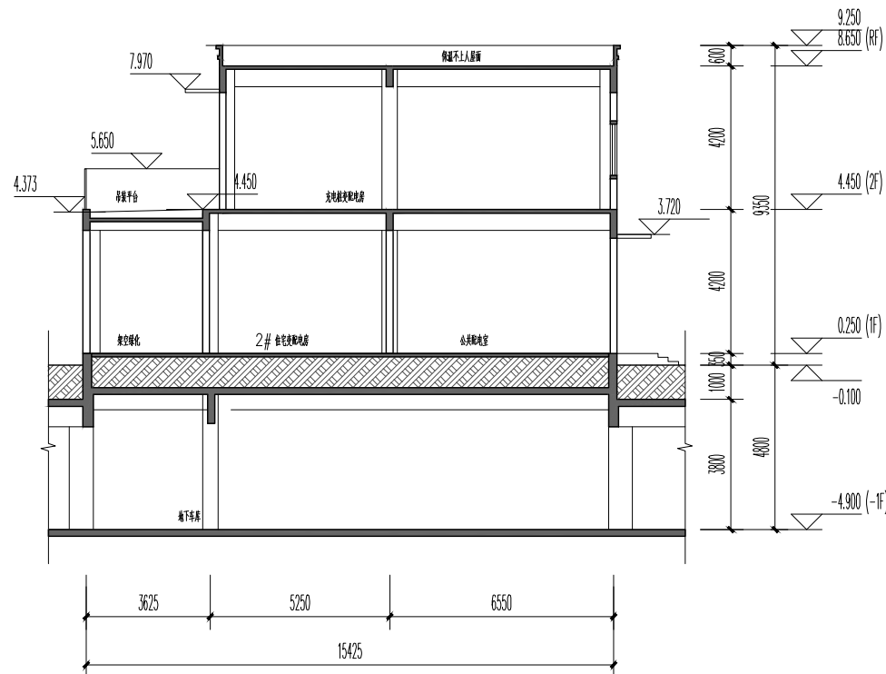
1-1剖面图
