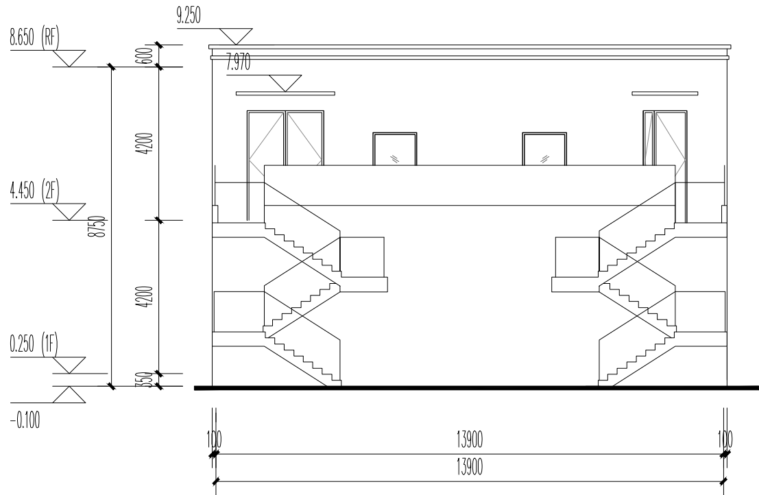
③~①轴立面图
