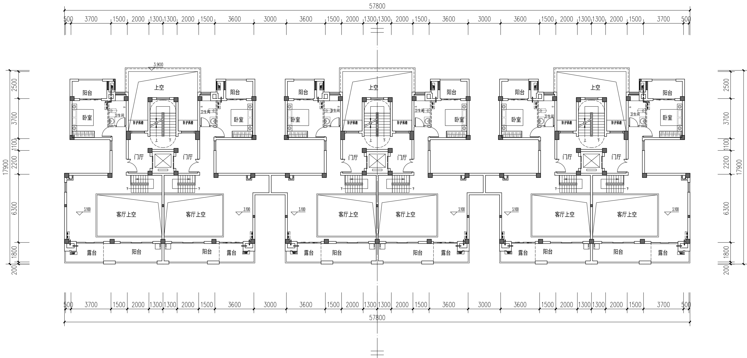
8#楼二层平面图
