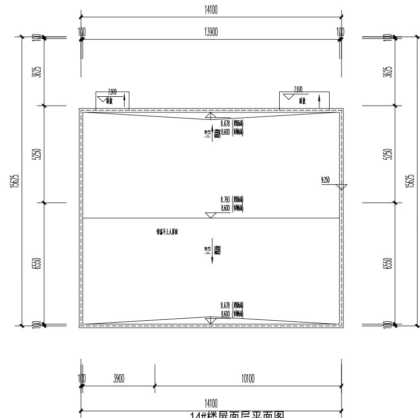
14#楼屋面层平面图
